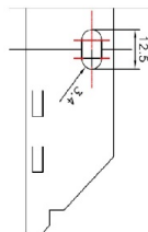
Detalle de uno de los orificios de anclaje (mm)
